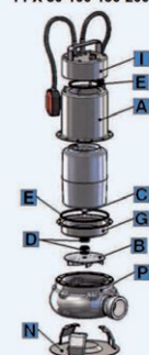
FPX 80-100-150-200
